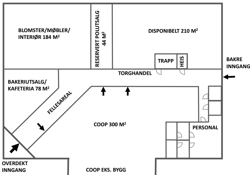
Planløsning for Vegglisenteret, byggetrinn 1
