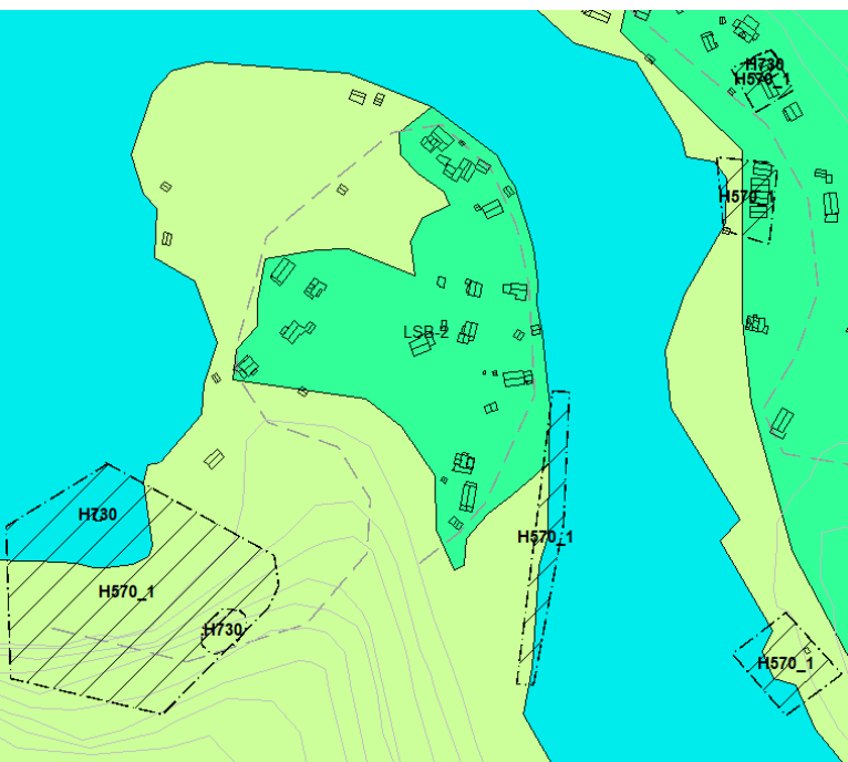
Figur 44: Døme på framstilling av freda kulturminne og verna kulturmiljø i plankartet. «H730» er freda kulturminne ved Skipshelleren, medan «H570» er angitt omsynssone for vern av kulturmiljøet i kontekst.
