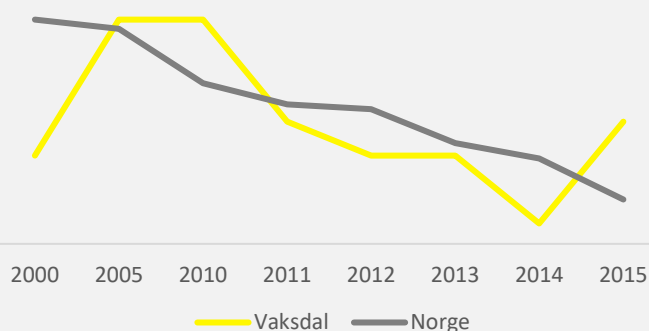
Figur 17: Relativ utvikling i tal trafikkulykker sidan år 2000
